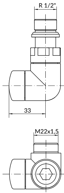
Winkeleck-Absperrventil
