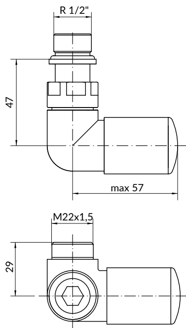
Winkeleck-Regelventil
